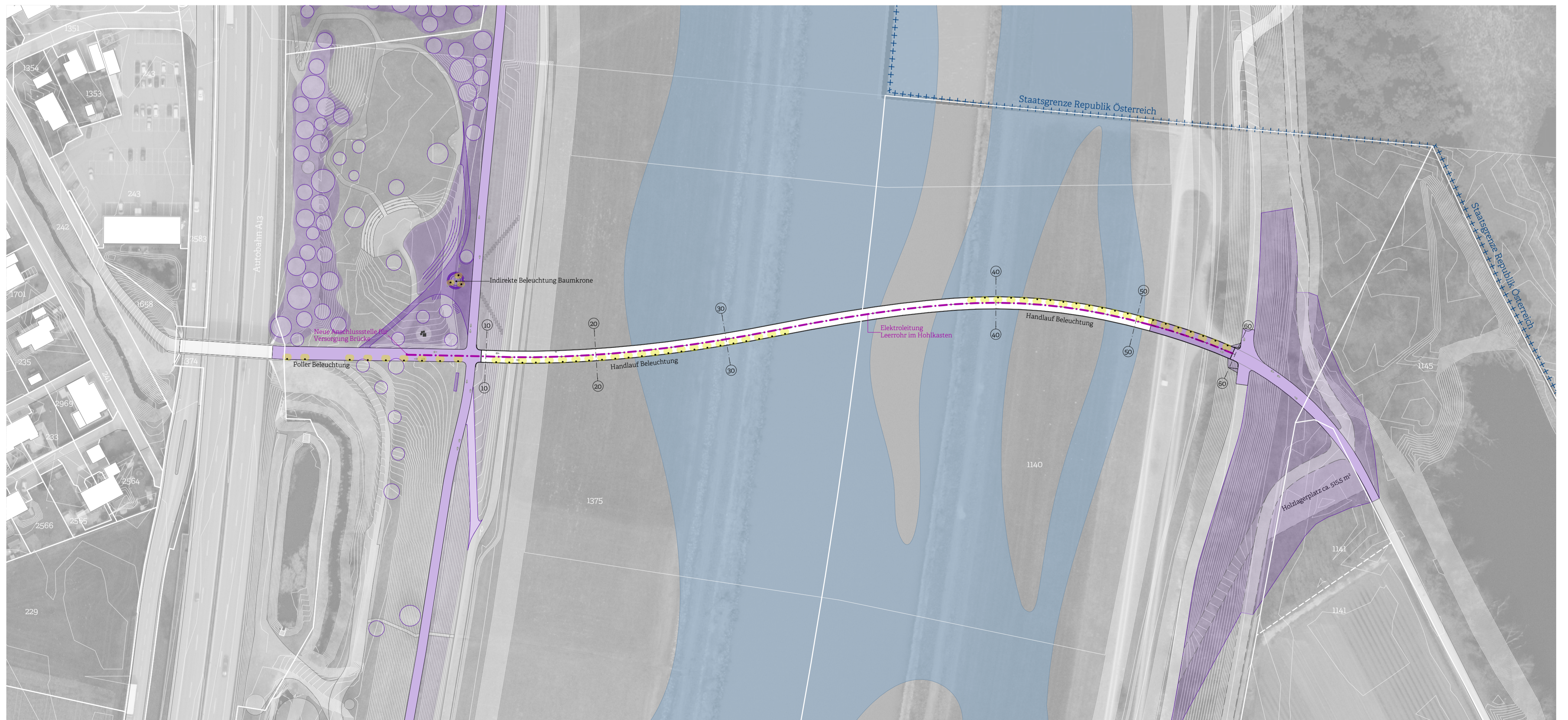
Beleuchtungskonzept - nach Rhesi M 1:1000
