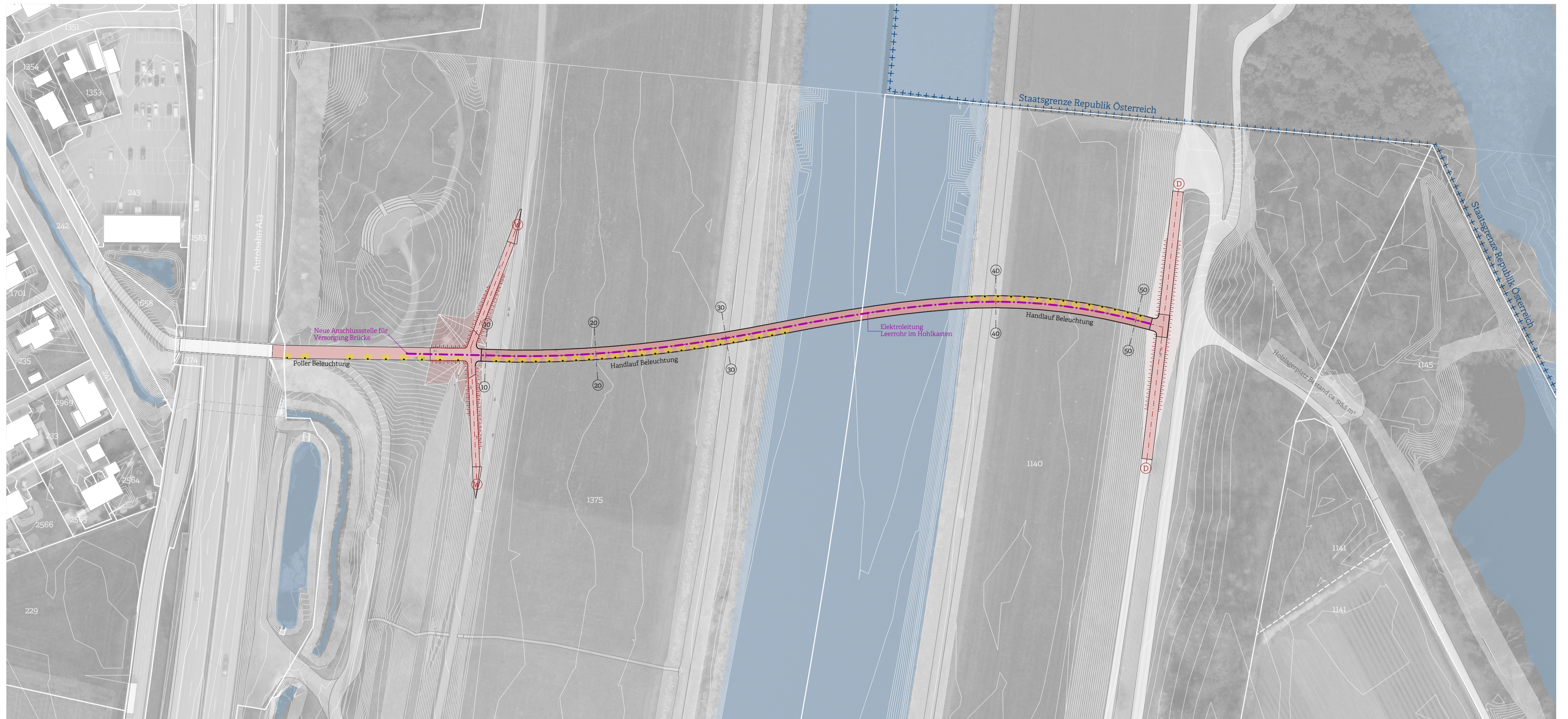
Beleuchtungskonzept - vor Rhesi M 1:1000
